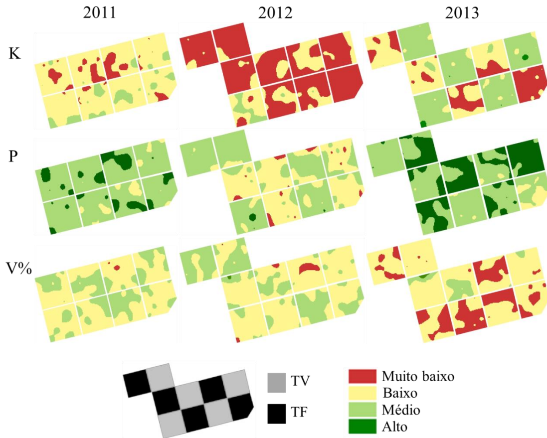
FIGURA 2. Mapas de K, P e V% do solo obtidos por meio de amostragem em grade
